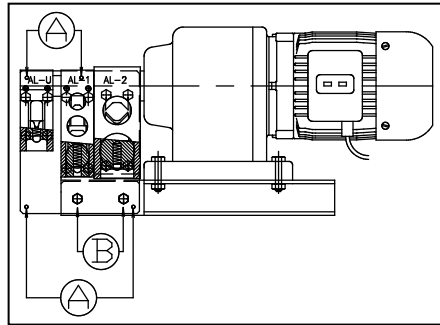
Abbildung 7.3-1: Ersetzen von Schneiddorn und/oder Feder 1 (dargestellt ist der AL1-2U)
