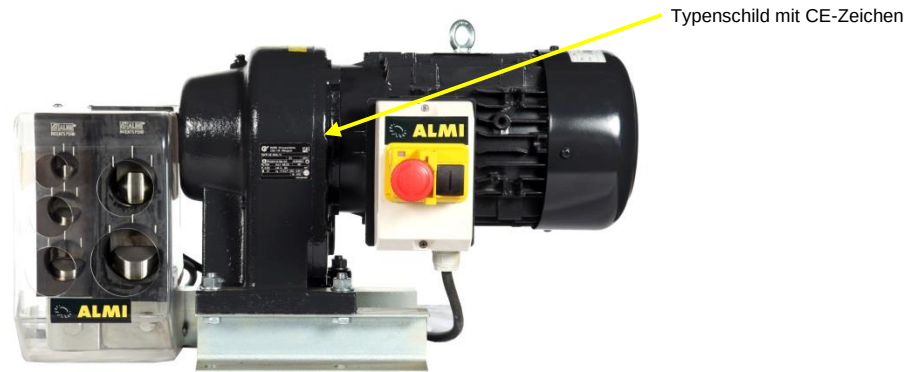
Abbildung 2.3-2: Befestigungsstelle des Typenschilds
