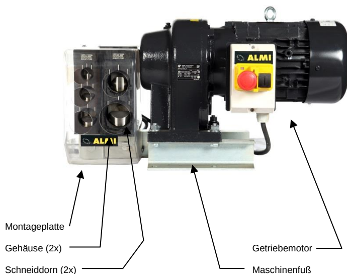
Abbildung 4.2-1: Aufbau der Maschine (dargestellt ist der AL1-2U)
