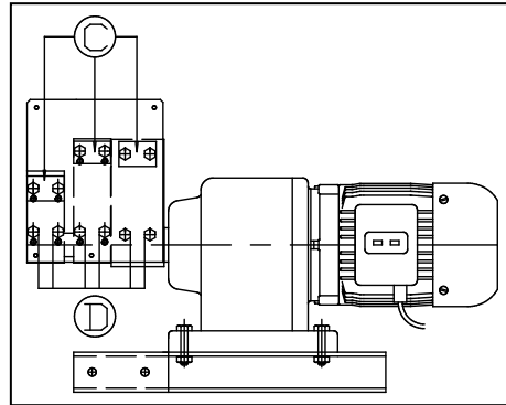
Abbildung 7.3-2: Ersetzen von Schneiddorn und/oder Feder 2 (dargestellt ist der AL1-2U)
